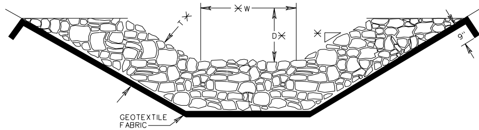
TYPE I RIPRAP DITCH PROTECTION
