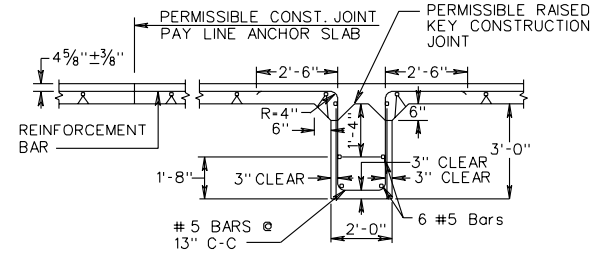
SECTION D-D
