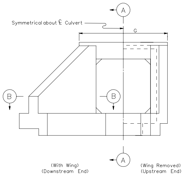
END ELEVATION
