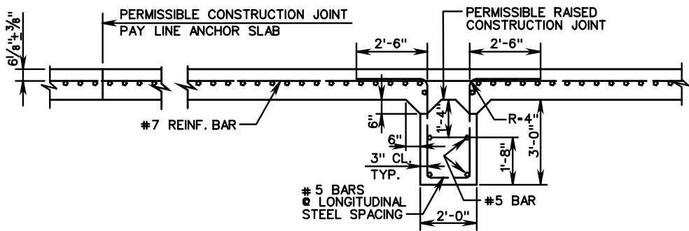
SECTION D-D
