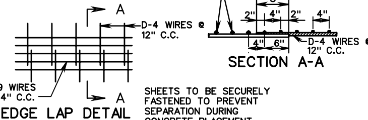
EDGE LAP DETAIL
