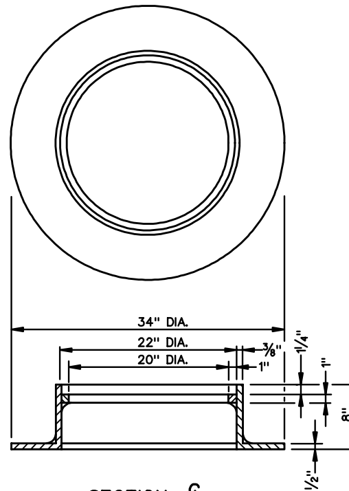
SECTION C-C MANHOLE FRAME
