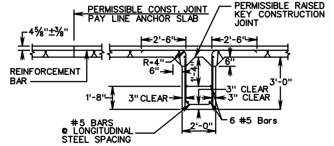
SECTION D-D
