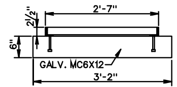
SECTION D-D
