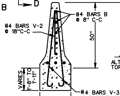
SECTION D-D
