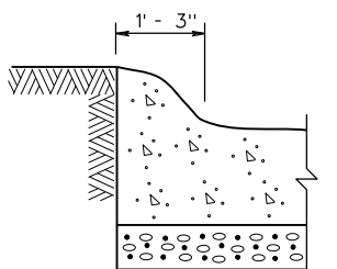
SECTION D-D
