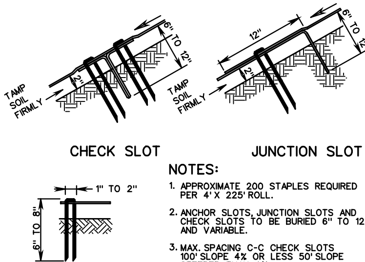
JUTE MESH
