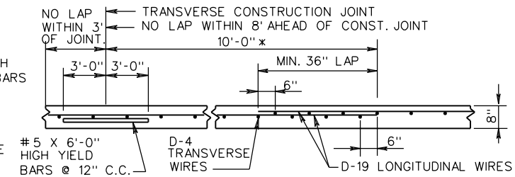
LONGITUDINAL SECTION
